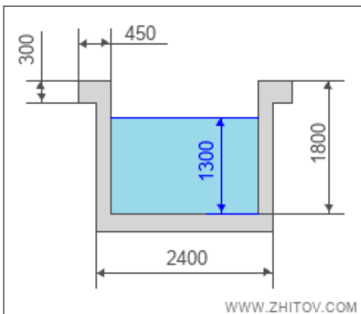
बेसिन आयाम - फ्रंट दृश्य
