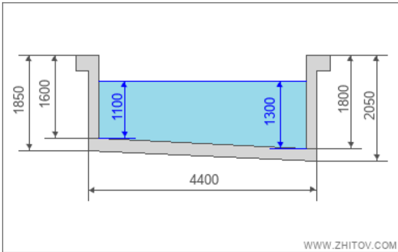
बेसिन आयाम - साइड दृश्य
