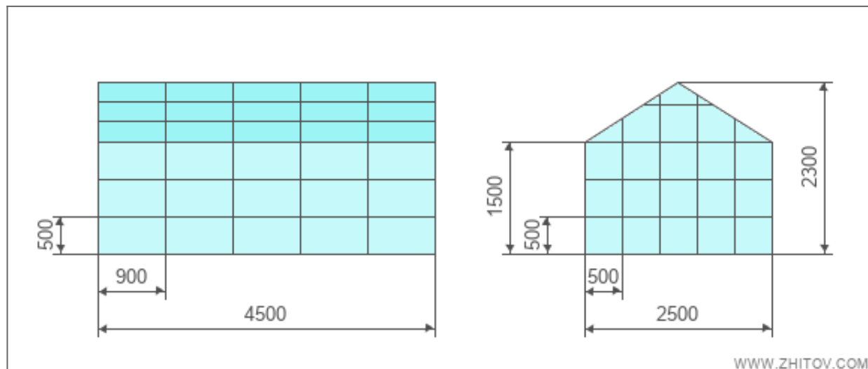
Вид сбоку и спереди
