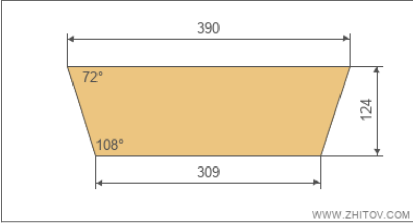
Detay çizimi
