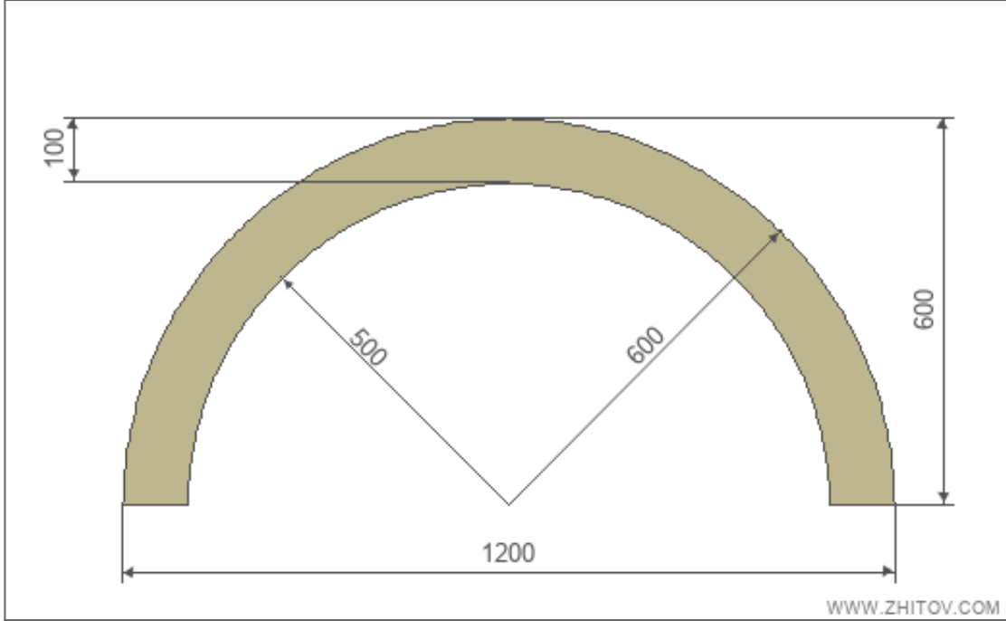
Kemerçizimi
